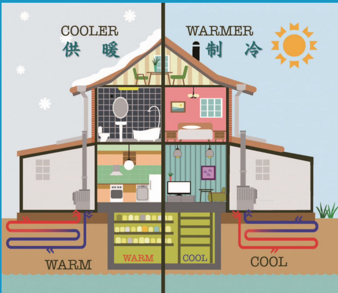
地源熱泵供暖製冷簡單示意圖
