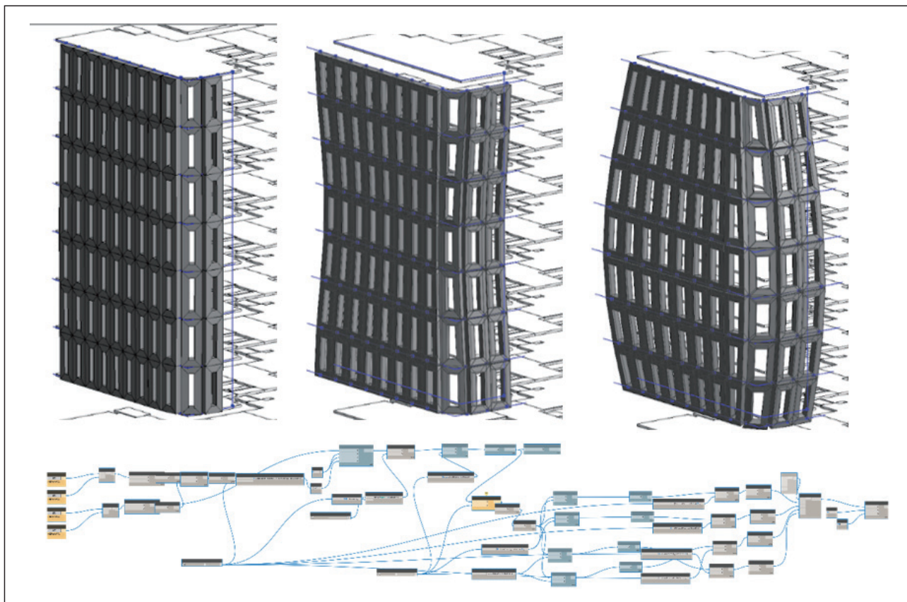
圖一：Revit & Dynamo 即時視覺參數化設計案例（帷幕造型參數化設計）
